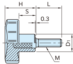
SFK SFK-SUS (Stud)
