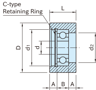
GRL-S-F (Steel)
