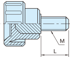
FTK FTK-SUS (Stud)
