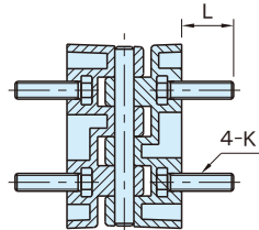
EMH-TT (Stud)
