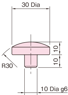
BJ733-10100 Radius Tip
