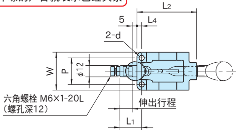
(夹紧时)
