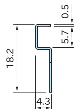
AMWD25-WS-B (2个1组)
