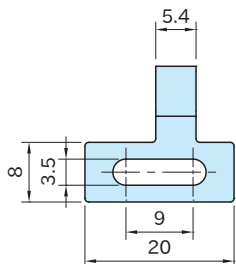
AMWD25-WS-B (2个1组)
