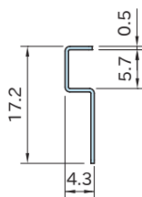
AMWD16-WS-B (2个1组)
