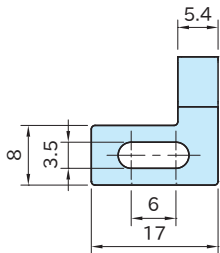
AMWD16-WS-B (2个1组)
